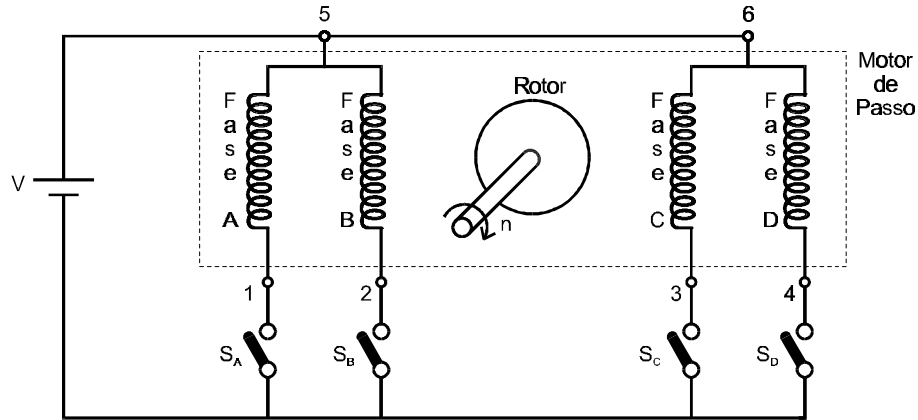
( a ) Circuito Simplificado de Acionamento
