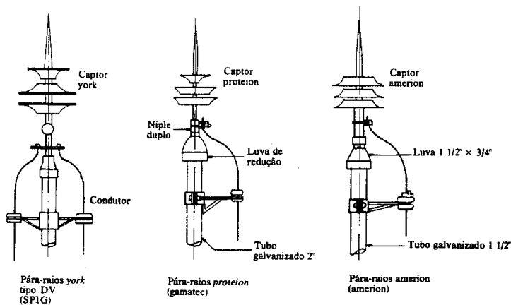
Captores de pára-raios radioativos
