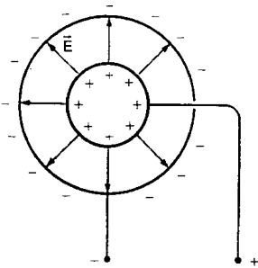
Capacitor esférico.
